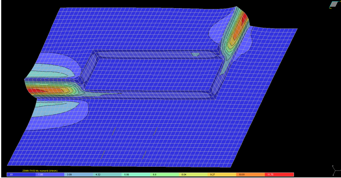
My zemin itki momenti
