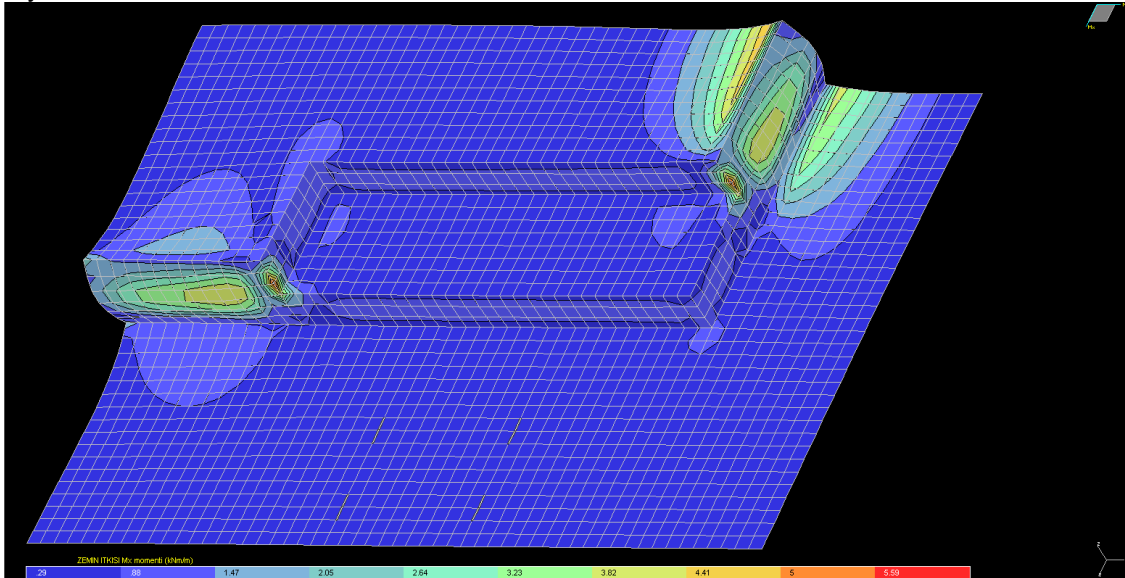
Mx zemin itki momenti
