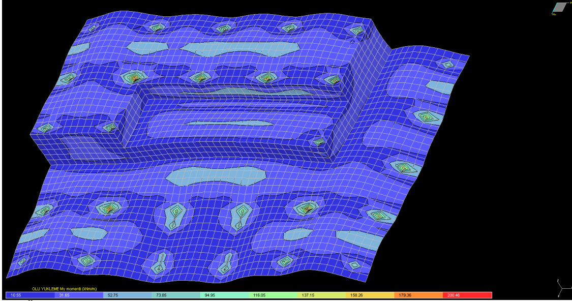
Mg Ölü yük momenti
